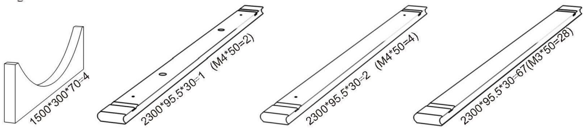
1 Cradles
